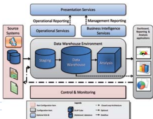
De referentiearchitectuur van onze softwareontwikkelstraat Endeavour BI.
